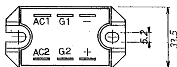
外形寸法図 OUTLINE DRAWING
