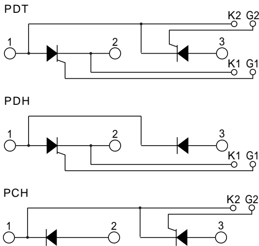
回路図 CIRCUIT
