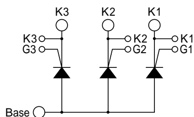
回路図 CIRCUIT
