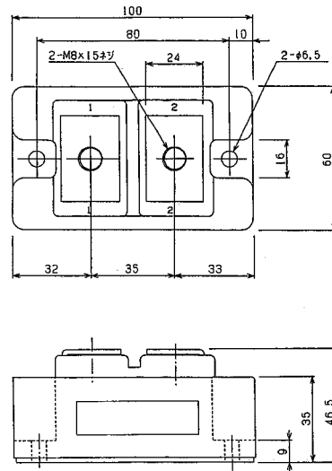
外形寸法図 OUTLINE DRAWING (単位 Dimension : mm)
