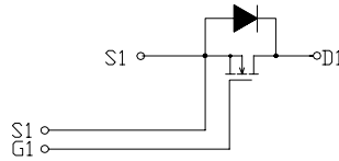
結線図
