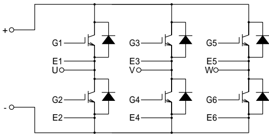
回路図 CIRCUIT
