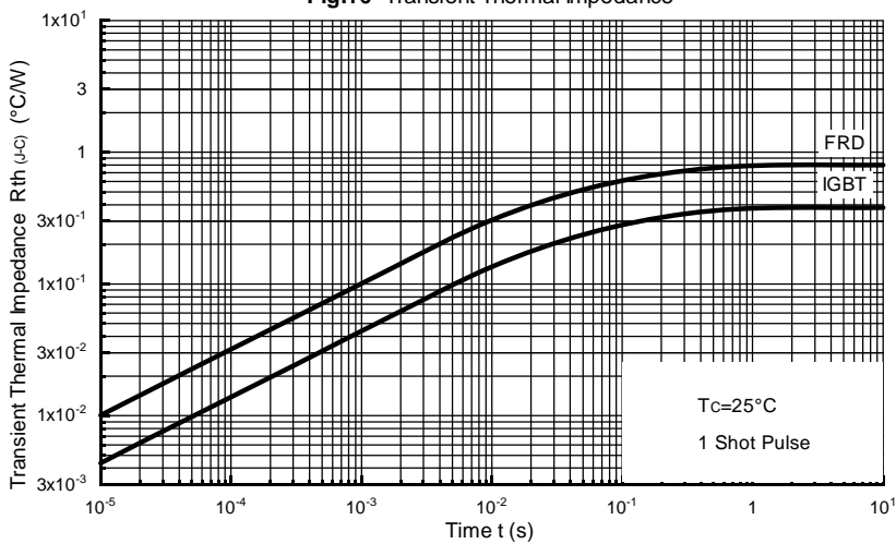
Fig.16- Transient Thermal Impedance
